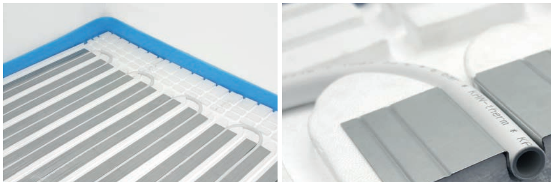
Рис. 36. Плита KAN-therm TBS 14 со стальным излучающим профилем
