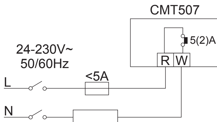
Рис. 65. Схема подключения клемм регулятора с еженедельным программатором 24 – 230 В к клеммной колодке Basic
