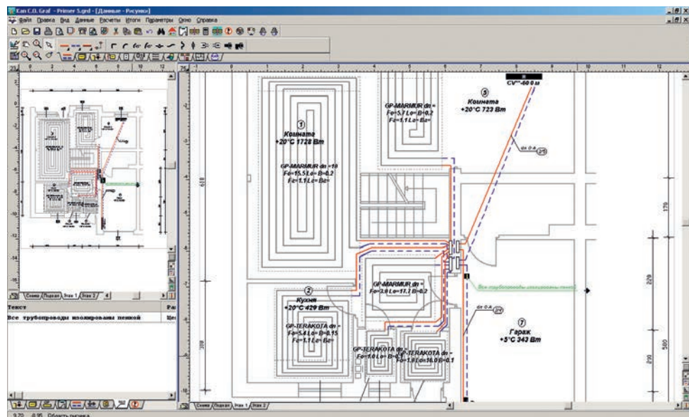
Рис. 81. План этажа с нанесенными подпольными отопительными приборами.
