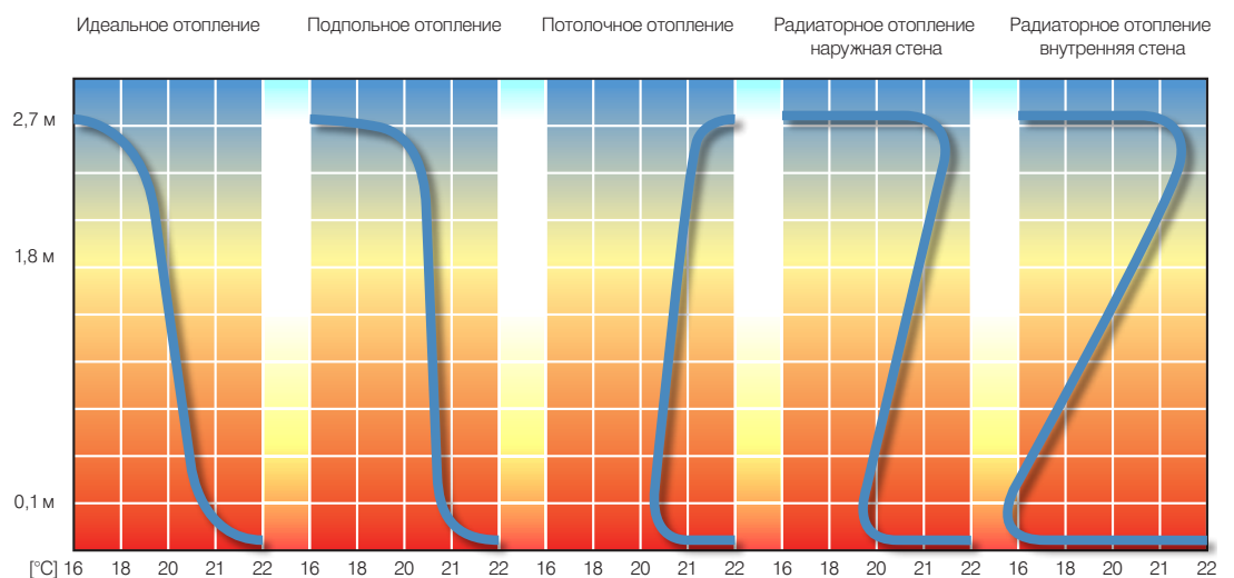
Рис. 1. Вертикальное распределение температуры для разных типов отопления
