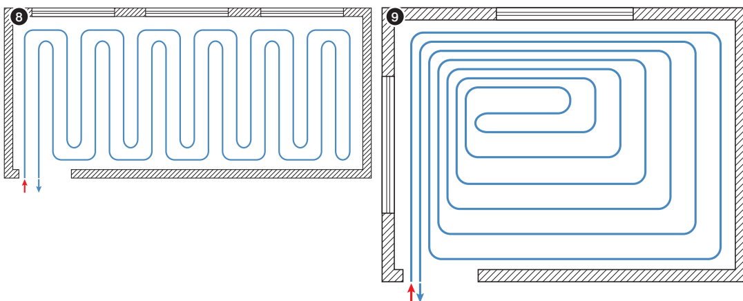
Рис. 8. Контур подпольного отопления/охлаждения в смешанной форме: вдвойный меандр.
