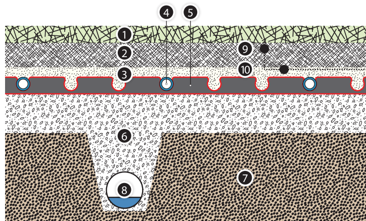
Рис. 45. Футбольное поле – искусственное покрытие
