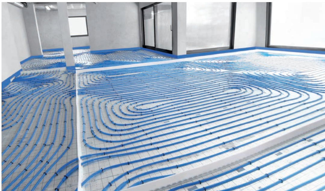
Рис. 24. Подпольное отопление, выполненное в системе KAN-therm Tacker
