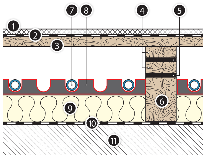
Рис. 38. Конструкция спортивного поверхностно-эластичного пола с системой подпольного отопления, выполненного из элементов системы KAN-therm Rail.
