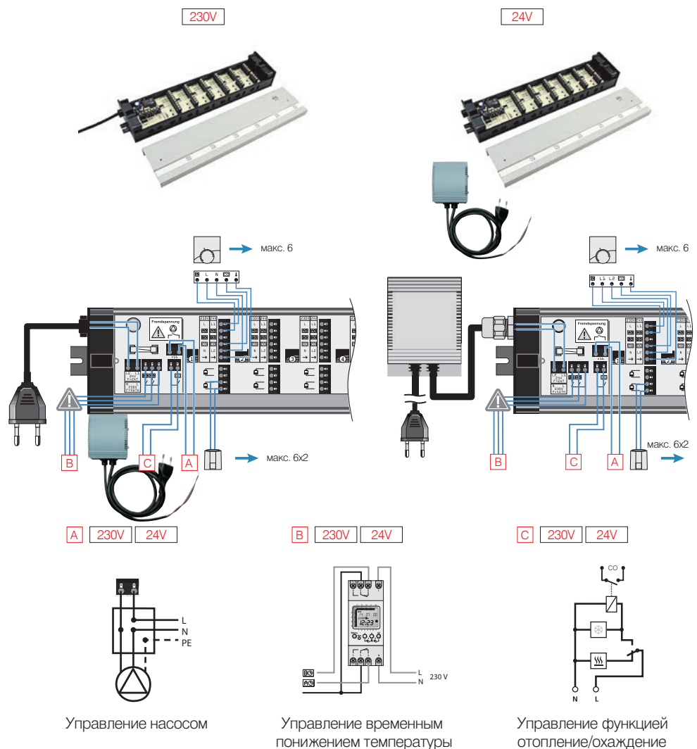
Рис. 71. Конфигурация клеммной колодки Basic 230 В или 24 В отопление/охлаждение с насосным модулем
