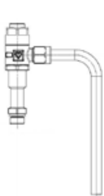
ГЕРЦ-пробоотборный клапан, возможно короткое и длинное исполнение
