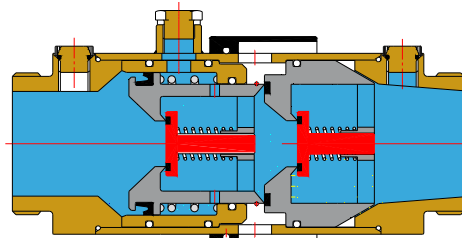
Системный разделитель под рабочим давлением, водоразбор отсутствует
