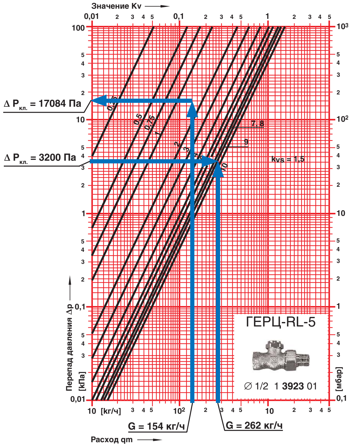
Рис. 7.9.: Пример определения гидравлических характеристик балансового вентиля ГЕРЦ-RL-5 для ветки «А» ( G_{уч.} = 262 кг/ч) и для ветки «Е» ( G_{уч.} = 154 кг/ч)
