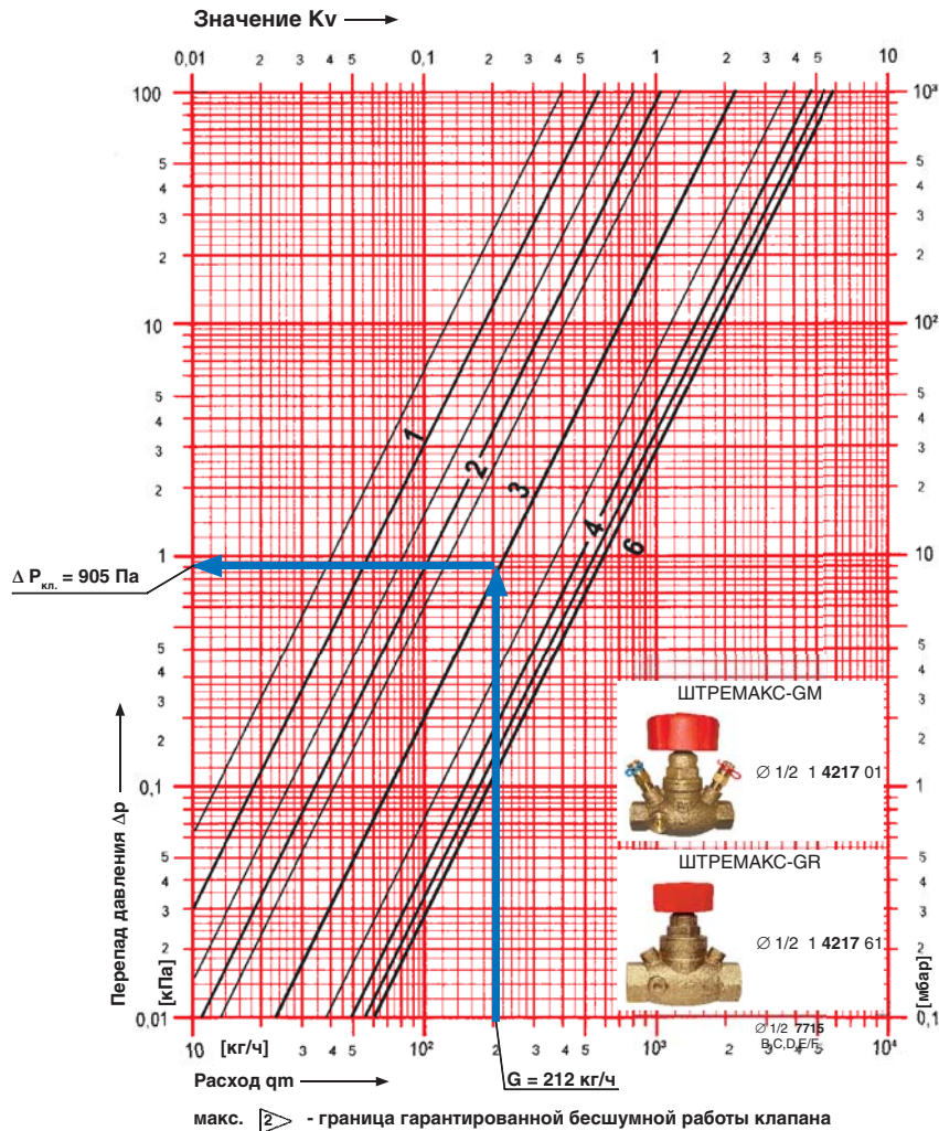
Рис. 7.5.: Пример определения \Delta P_{\text{кл}} балансового вентиля ШТРЕМАКС-GM, устанавливаемого на Ст.13 ( G_{\text{уч.}} = 212 \text{ кг/ч} , \Delta P_{\text{кл.}} = 905 \text{ Па} , k_v = 2,2 \text{ м}^3/\text{ч} )
